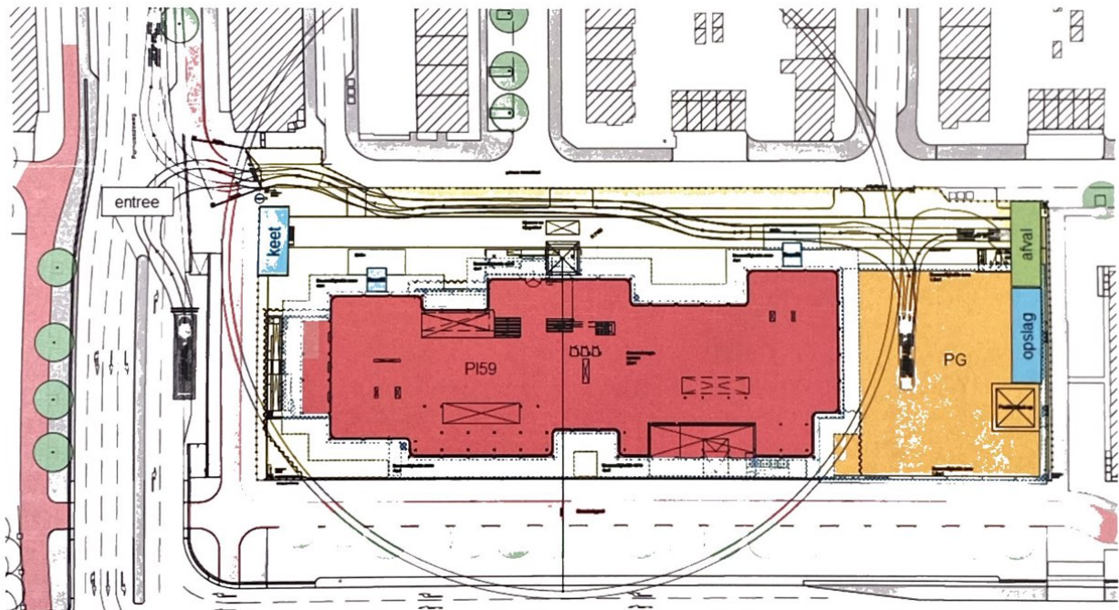
afbeelding 2; bouwplaatsinrichting
